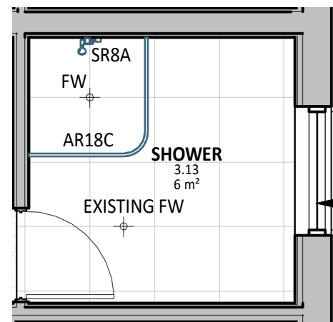
16 PLAN DETAIL 1 : 50
