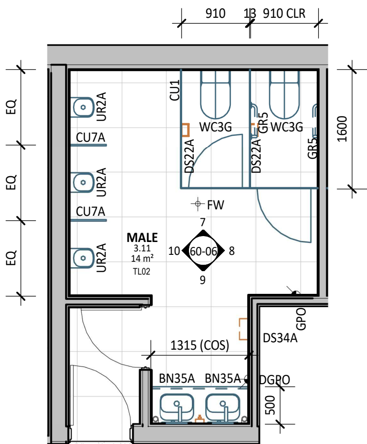
6 PLAN DETAIL 1 : 50
