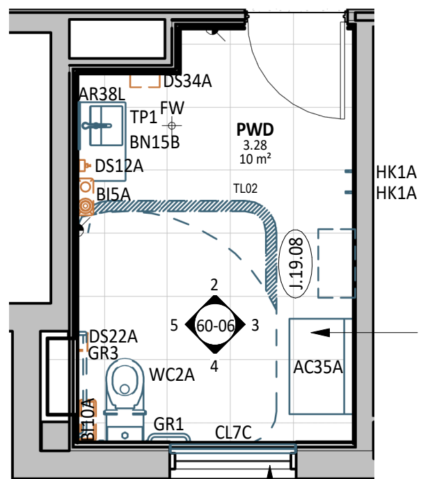
1 PLAN DETAIL 1 : 50
