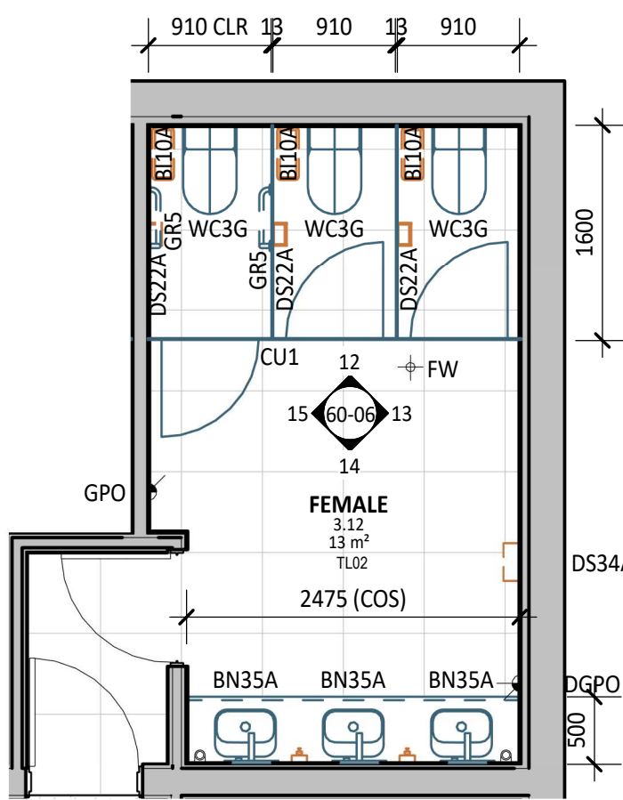
11 PLAN DETAIL 1 : 50
